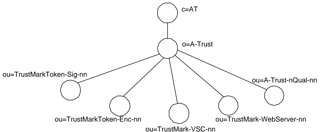
Abbildung 2 A-Trust Verzeichnisbaum
